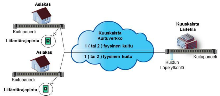
Kuva: Tilaajakuituyhteys
